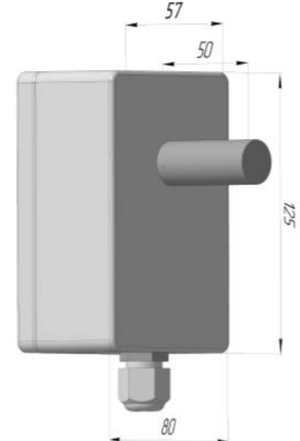
Рис.2 Габаритные размеры
